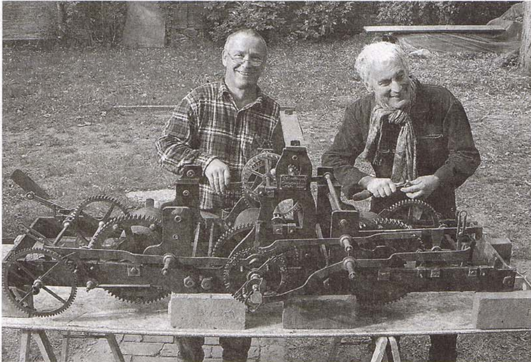
Der Uhrmacher Ulrich Frank aus Görne und der Vicheler Detlef Schnabel haben in mehreren hundert Arbeitsstunden die Vicheler Kirchturmuhre restauriert und dabei einen wahren Schatz neu belebt: eine dreiteilige Moellinger-Kirchturmuhre aus dem Jahre 1868. Fotos: privat
